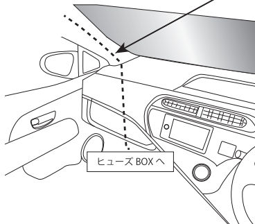
オプション品＝常時電源ケーブル（MA2）
