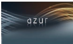
起動画面
